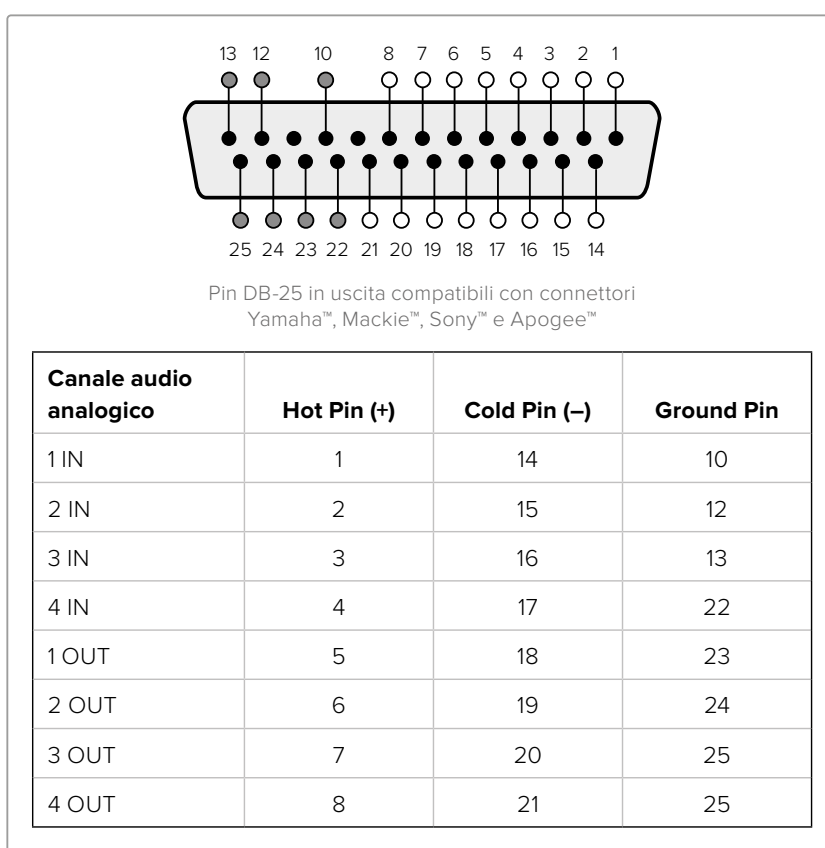
Piedinatura per audio analogico su Teranex 2D
