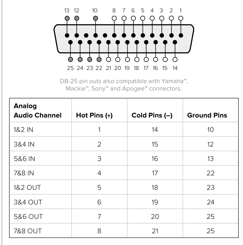
Teranex 2D İşemci AES/EBU ses pim bağlantıları
