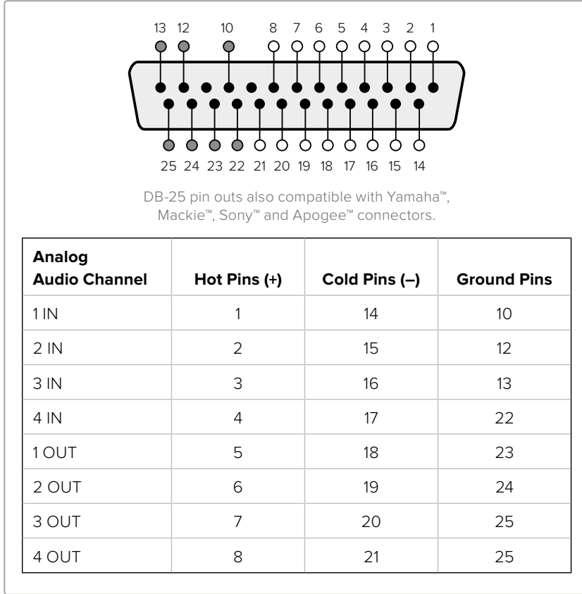
Teranex 2D İşlemci analog ses pim bağlantıları
