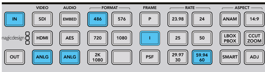
按IN按钮可让控制面板按钮显示输入格式。 在上图中,输入格式为486i59.94,通过模拟分量接口,并带模拟音频信号。
