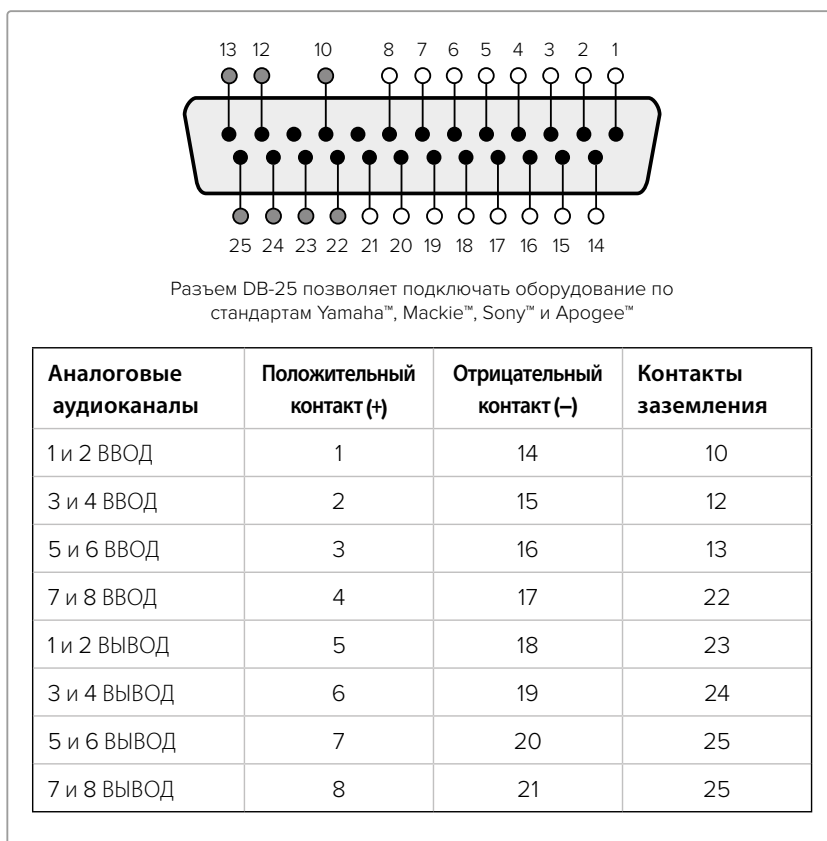
Схема каналов AES/EBU-звука (Teranex 2D)
