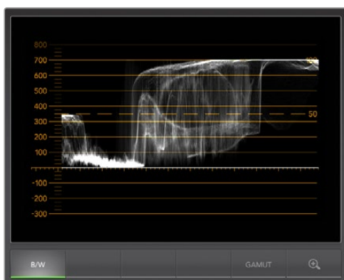
Monitor de Forma de Onda.
