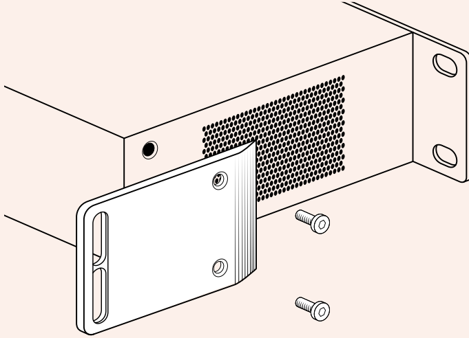
Kutuda gelen koruyucuları Teranex AV'nizin her iki tarafına takın.
