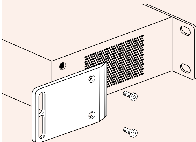
Installa le due protezioni antiurto serrando le viti sui due lati di Teranex AV
