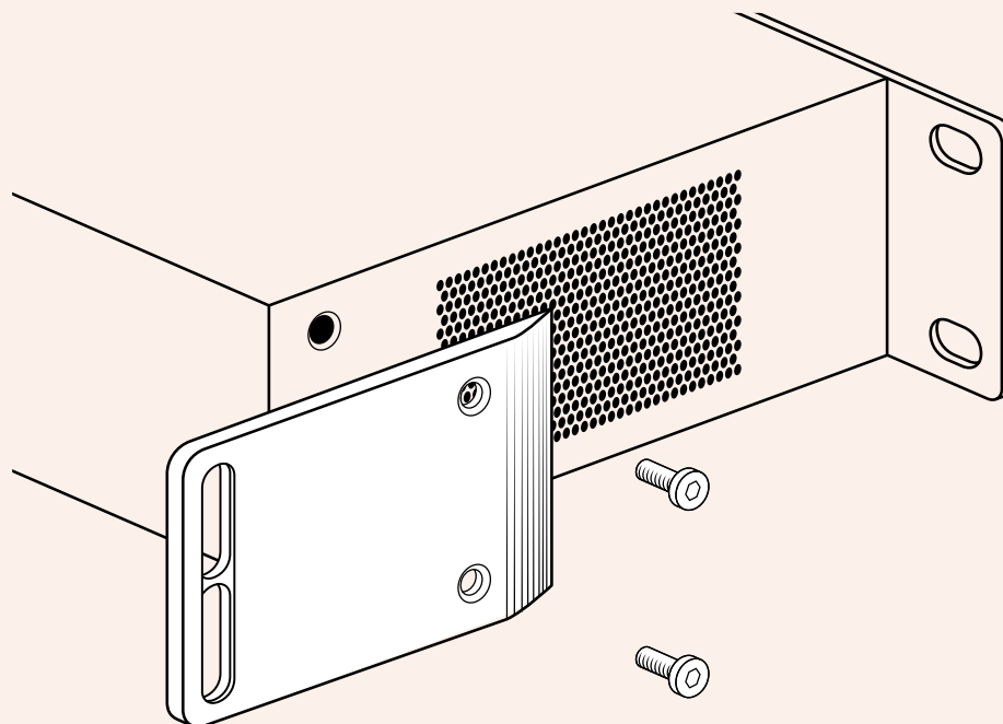
Зажимы для установки на Teranex AV по бокам корпуса
