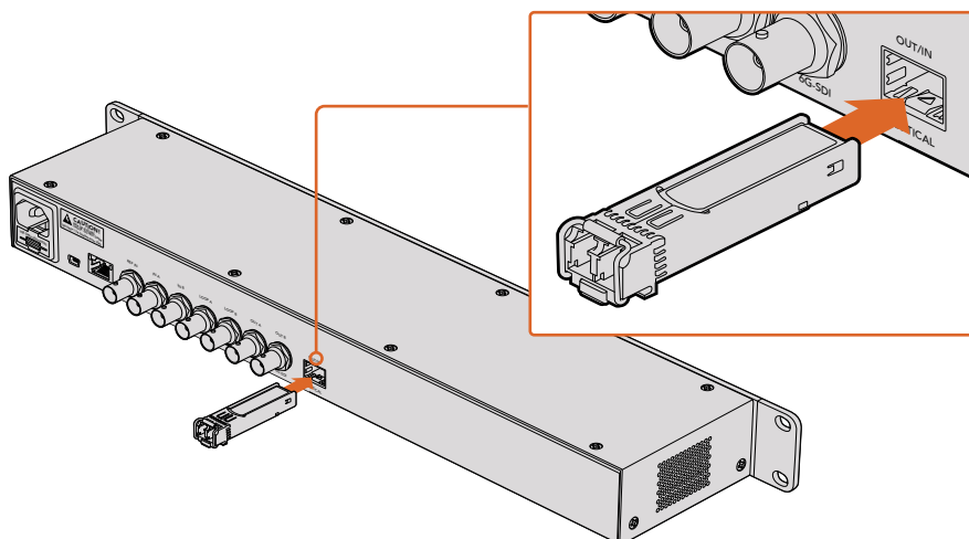
Installazione del modulo SFP su Teranex Express
