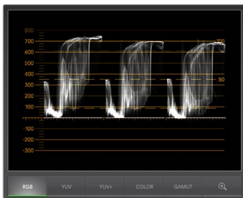
RGB 퍼레이드 보기
