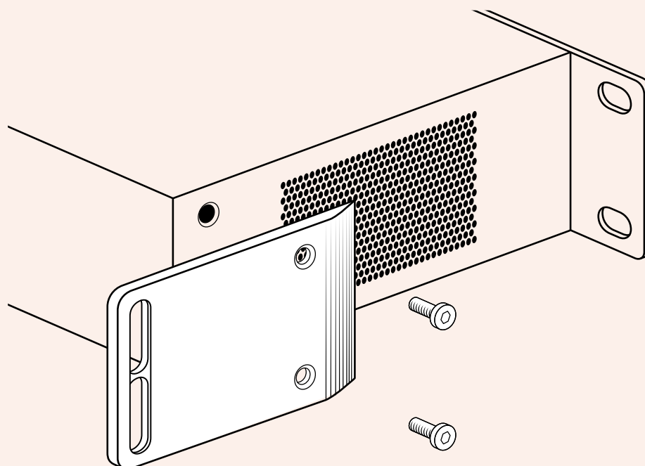
同梱のバンパーをTeranex AVの両再度に取り付けます。
