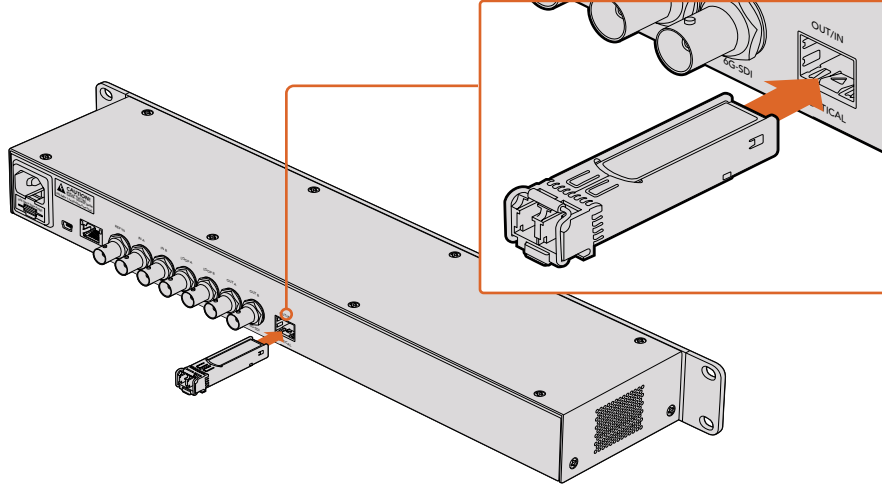
SFP modülünün Teranex Express cihazına takılması.
