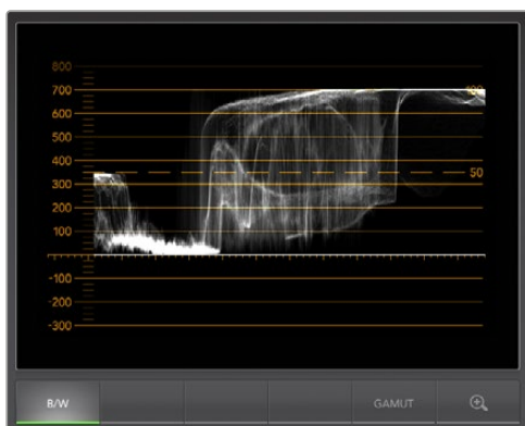
Affichage Forme d'onde
