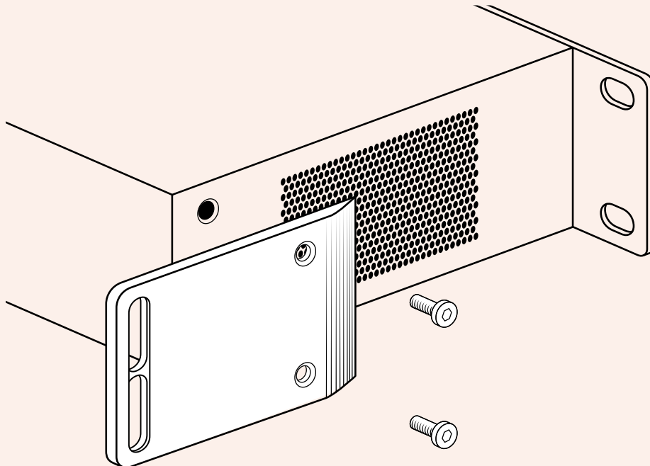
Sujete los paragolpes a los laterales de la unidad.
